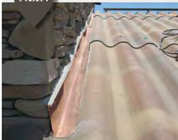
Im Bild ein Beispiel für falsche Installation.
